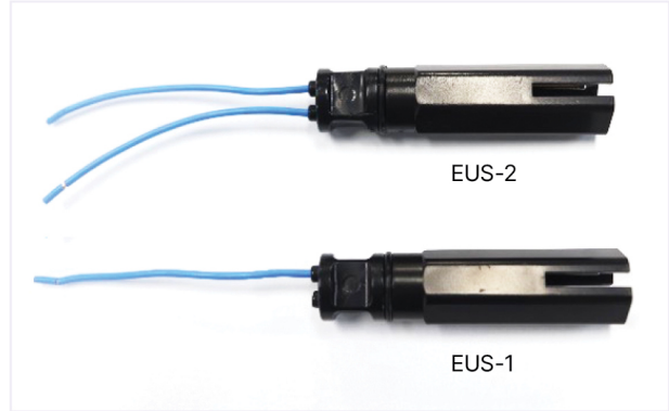
심정용 센서
